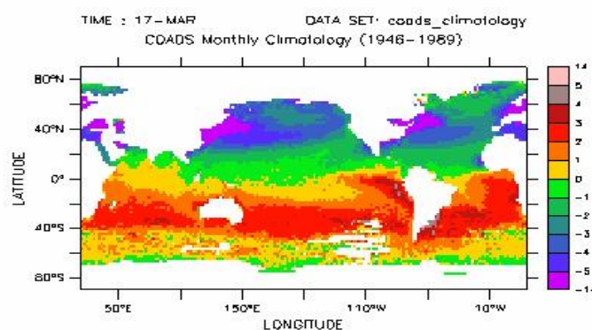
SST Anomaly
