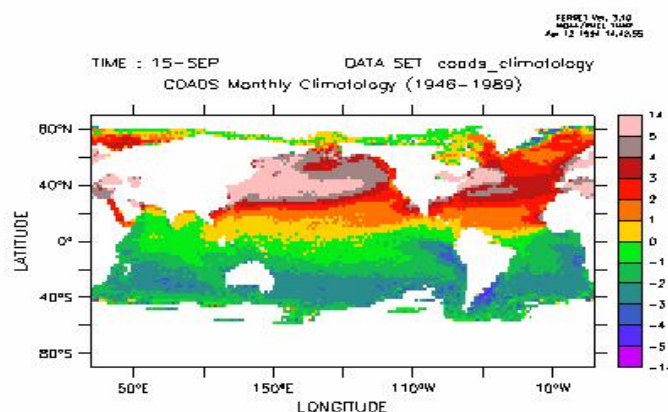
SST Anomaly
